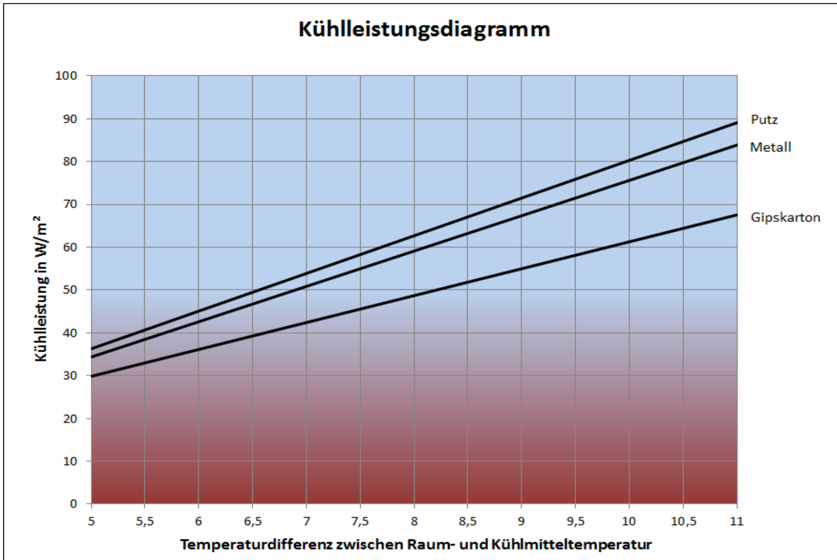
Spezifische Kühlleistung in Abhängigkeit vom Material
