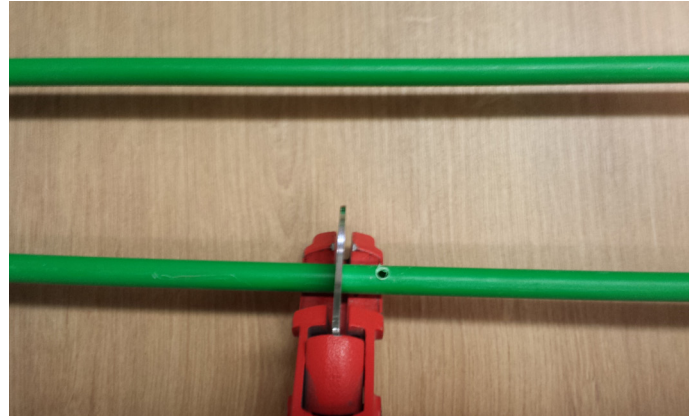
Beschädigte Stelle mit einer Rohrschere herausschneiden
