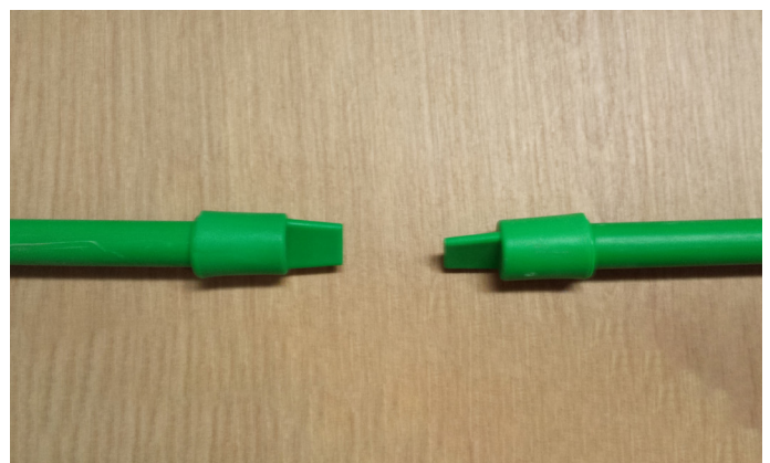
Mittels Reparaturdorn-Set und Außen-Stopfen beide Enden verschweißen
